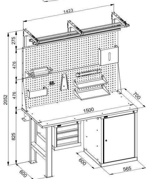
Верстак ДиКом ВЛ-150
