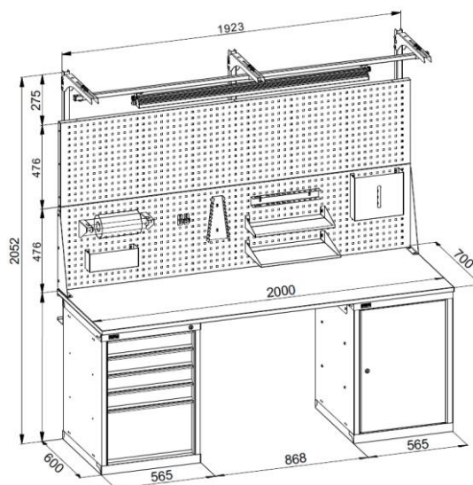
Верстак ДиКом ВЛ-200
