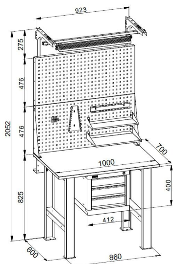
Верстак ДиКом ВЛ-100
