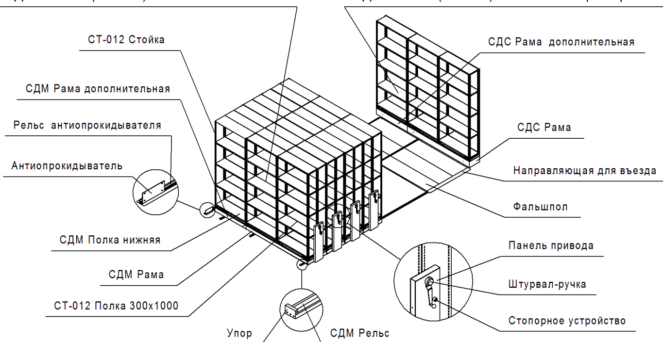
СДМ- 3 Рама(СТ-012) Стеллаж мобильный
