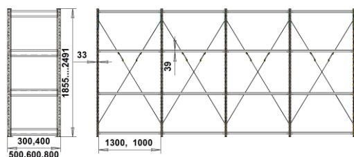
Схема вариантов установки стеллажа СТ-031
