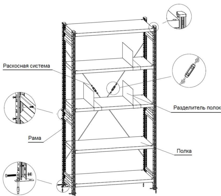
Схема вариантов установки стеллажа СТ-031
