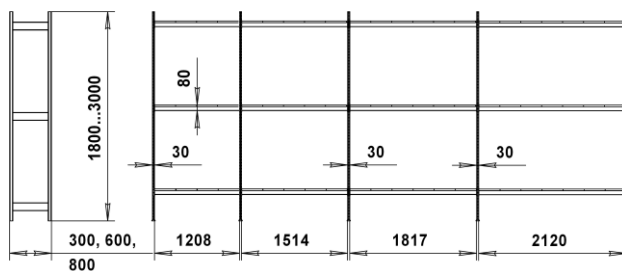
Схема вариантов установки стеллажа СТ-023
