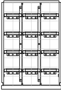
Типоразмер-003 Тумбы ВЛ-003 и ВС-003
